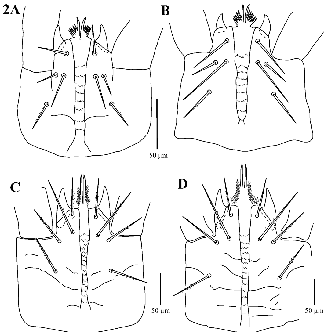
FIGURE 2. Euryparasitus deutonymphs, subcapitulum. A: E. occidentalis n. sp.; B: E. longicheta Bondartchuk & Buyakova; C: E. maseri n. sp.; D: E. calcarator (Banks).
