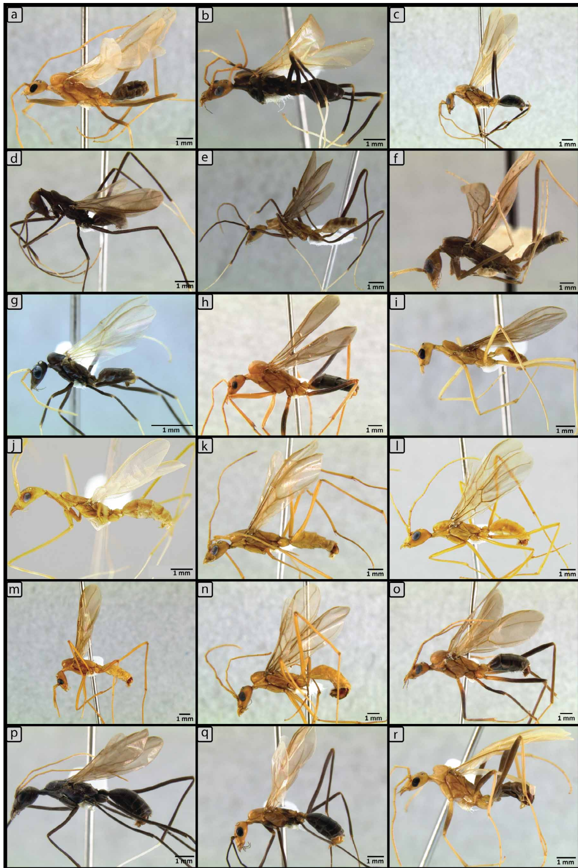
FIGURE 24. Macro- Leptomyraxes males: a) L. cnemidatus , b) L. darlingtoni , c) L. erythrocephalus , d) L. flavitarsus , e) L. fragilis , f) L. melanoticus , g) L. mjobergi , h) L. nigriventris , i) L. pallens , j) L. puberulus , k) L. rothneyi , l) L. ruficeps , m) L. rufipes , n) L. rufithorax , o) L. tibialis , p) L. unicolor , q) L. varians , r) L. wiburdi .
