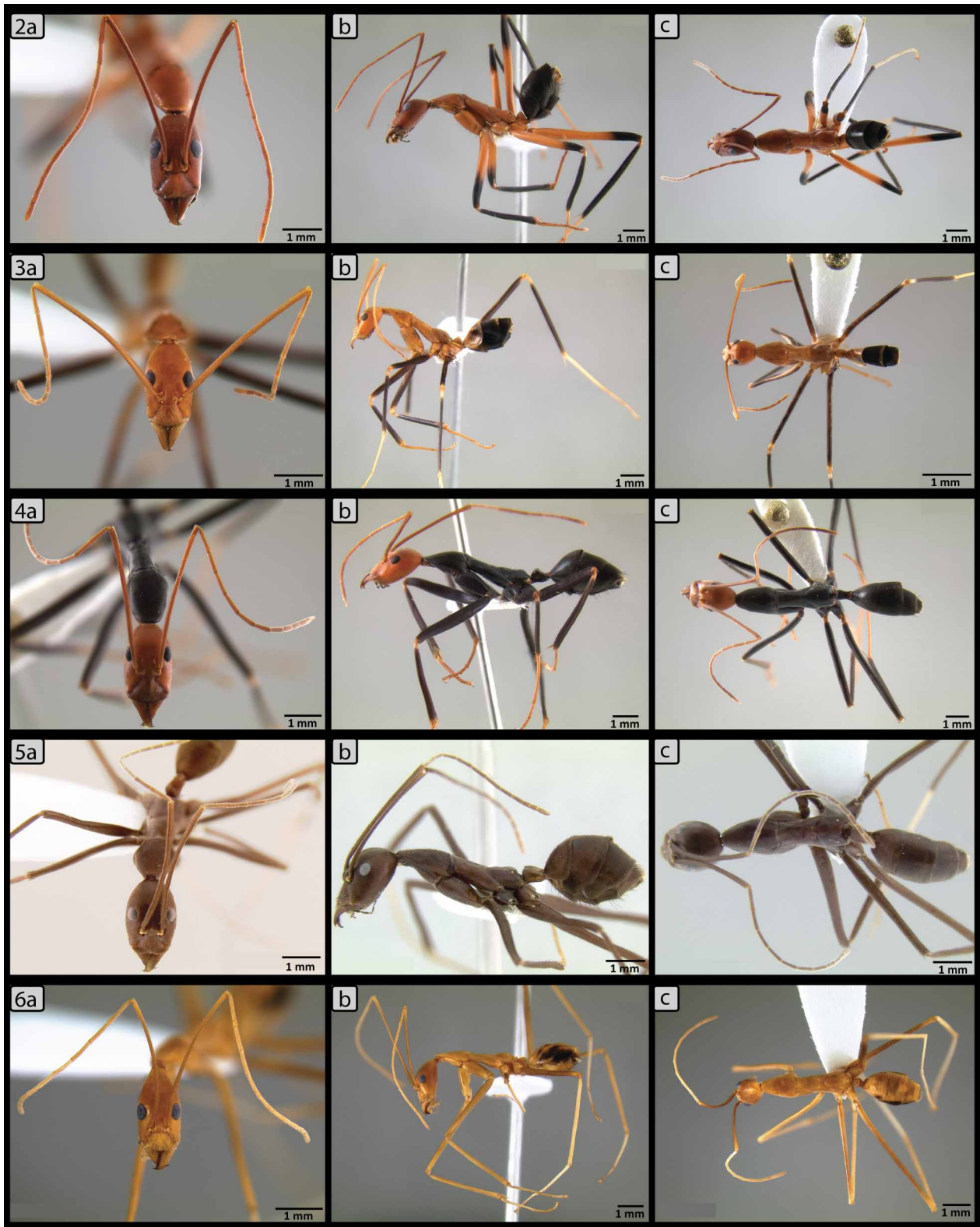
FIGURES 2–6. Macro- Leptomyrmex workers in head, profile and dorsal view. Fig. 2: L. cnemidatus . Fig. 3: L. darlingtoni . Fig. 4: L. erythrocephalus . Fig. 5: L. flavitarsus . Fig. 6: L. fragilis .
